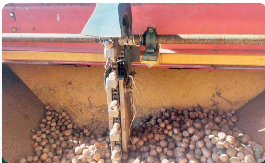
Makkvetőgép adagolóeleme
